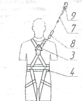
1 - ремень; 2 - пряжка ремня; 3 - кольцо (элемент крепления); 4 - кушак; 5 - лямка наплечная; 6 - лямка набедренная; 7 - гибкий элемент стропа; 8 - амортизатор; 9 - карабин (элемент соединительный)
